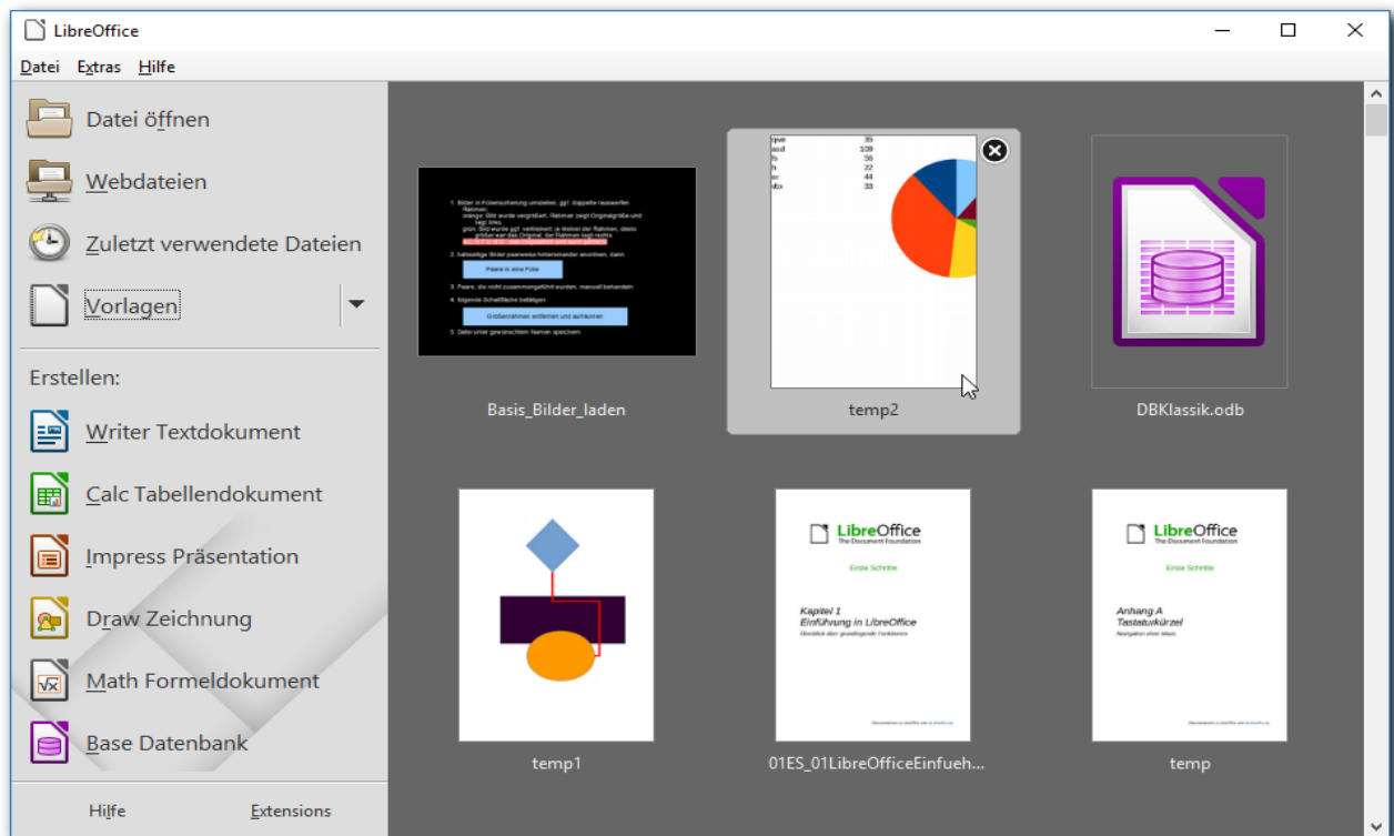
Abbildung 2: LibreOffice Startcenter
